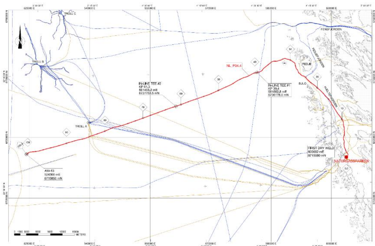
Figur 4-25: Rørledningstraseen fra mottaksterminal til injeksjonsbrønn i Aurora-lisensen.
